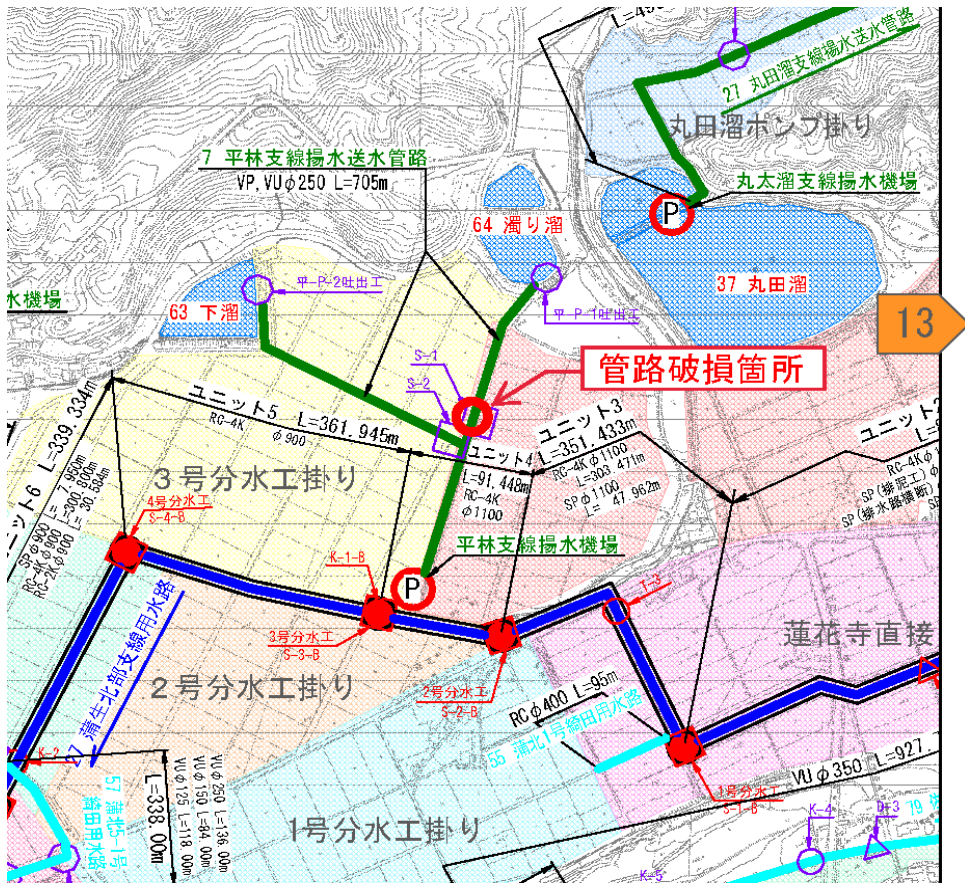
管路破損箇所 位置図
